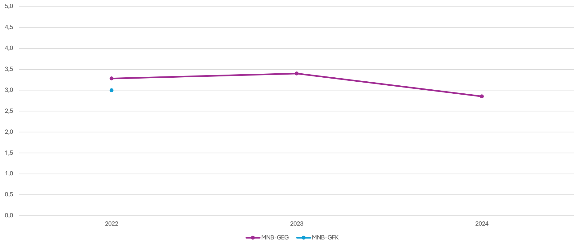
Snittkarakter studieprogram
