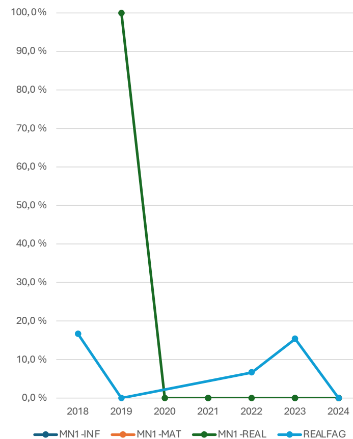
Strykprosent årsenheter
