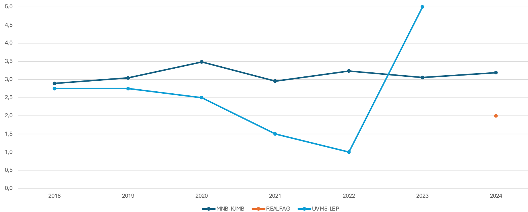
Snittkarakter studieprogram
