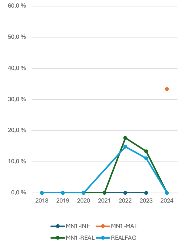
Strykprosent årsenheter
